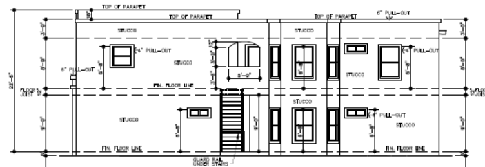
10. RIGHT ELEVATION
