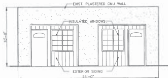
GARAGE CONVERSION ELEV. SCALE: 1/8"=1'-0"
